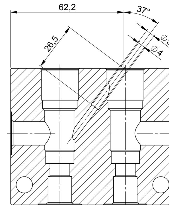
SEZIONE C-C
