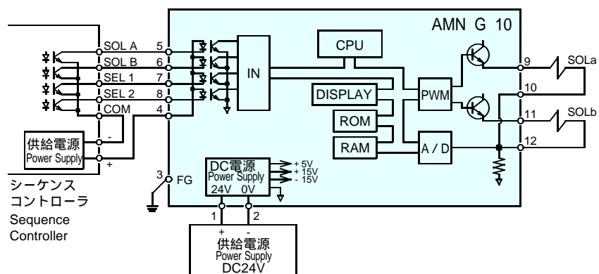
使用回路例 Example Diagram
