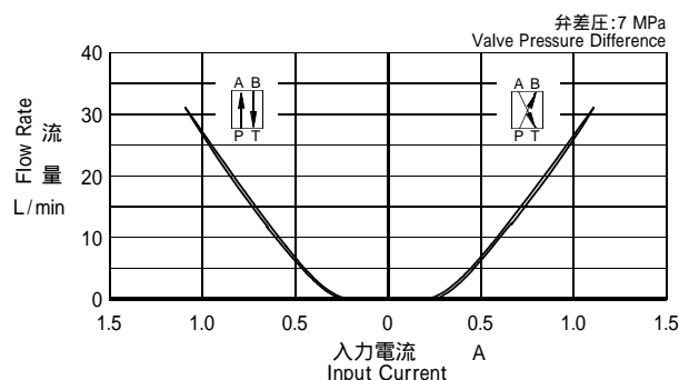
電流 - 流量特性 Input Current vs. Flow
